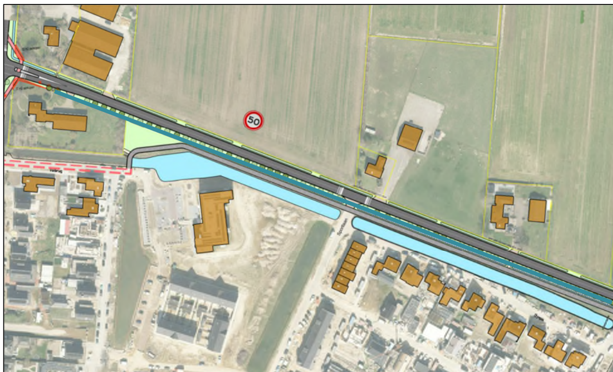
Figuur 3-4 Aanleg greppel. Vanaf de kruising tot aan de rotonde (Macharensesweg/Spitsbergerweg) dient ongeveer 98 m 3 aan waterberging gerealiseerd te worden. Echter vanaf de kruising (Spitsbergerweg/Oijensesweg) tot aan het begin van de blauwe streep is de berm niet breed genoeg voor een greppel.
