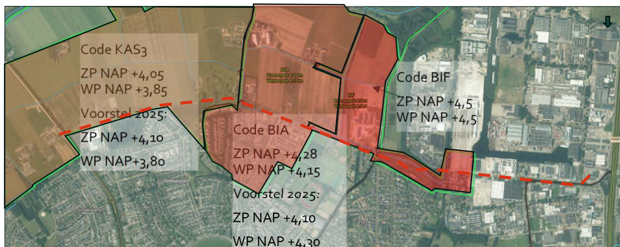
Figuur 2-3 Watersysteem projectlocatie Noordelijke ontsluitingsweg te Oss waarbij de verschillende peilgebieden met een zwarte lijn zijn aangegeven. De gegeven peilen betreffen het zomer- en winterpeil in de praktijk. De rood gestreepte lijn betreft de projectlocatie.
