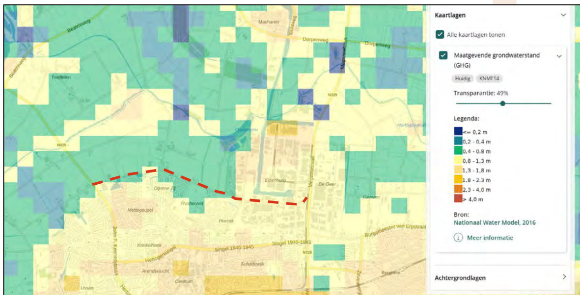
Figuur 2-7 Gemiddeld Hoogste Grondwaterstand (bron: Klimaat-effectatlas ). De gemiddeld hoogste grondwaterstand (GHG) zit op 0,4 à 0,8 m -mv. aan de westzijde van de projectlocatie en aan de oostzijde op 0,8 à 1,3 m -mv.
