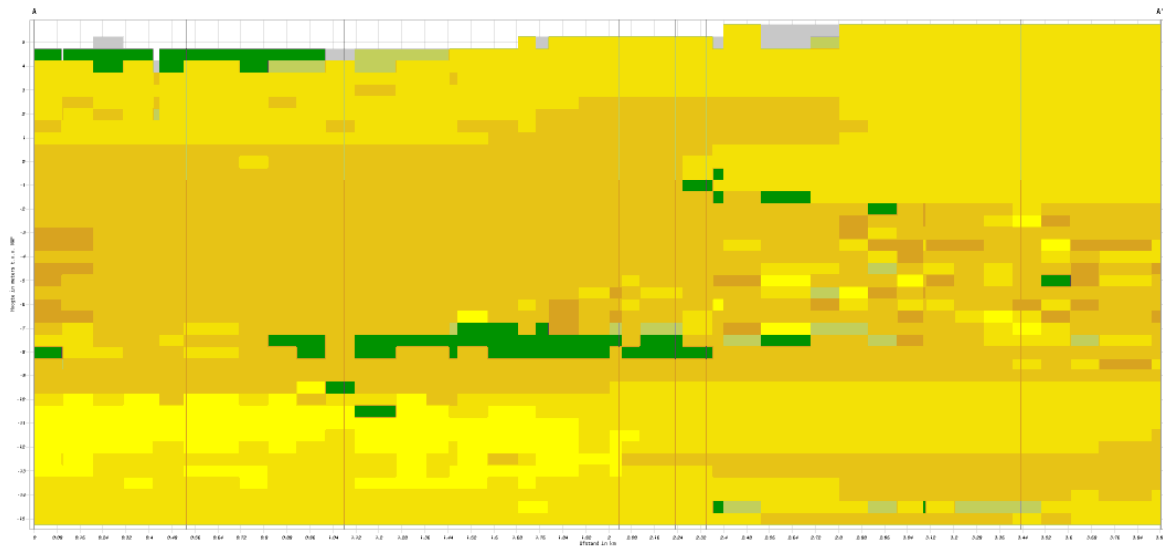
Figuur 2-4 Verticale doorsnede meest waarschijnlijke lithoklasse west-oost, projectlocatie Oss
