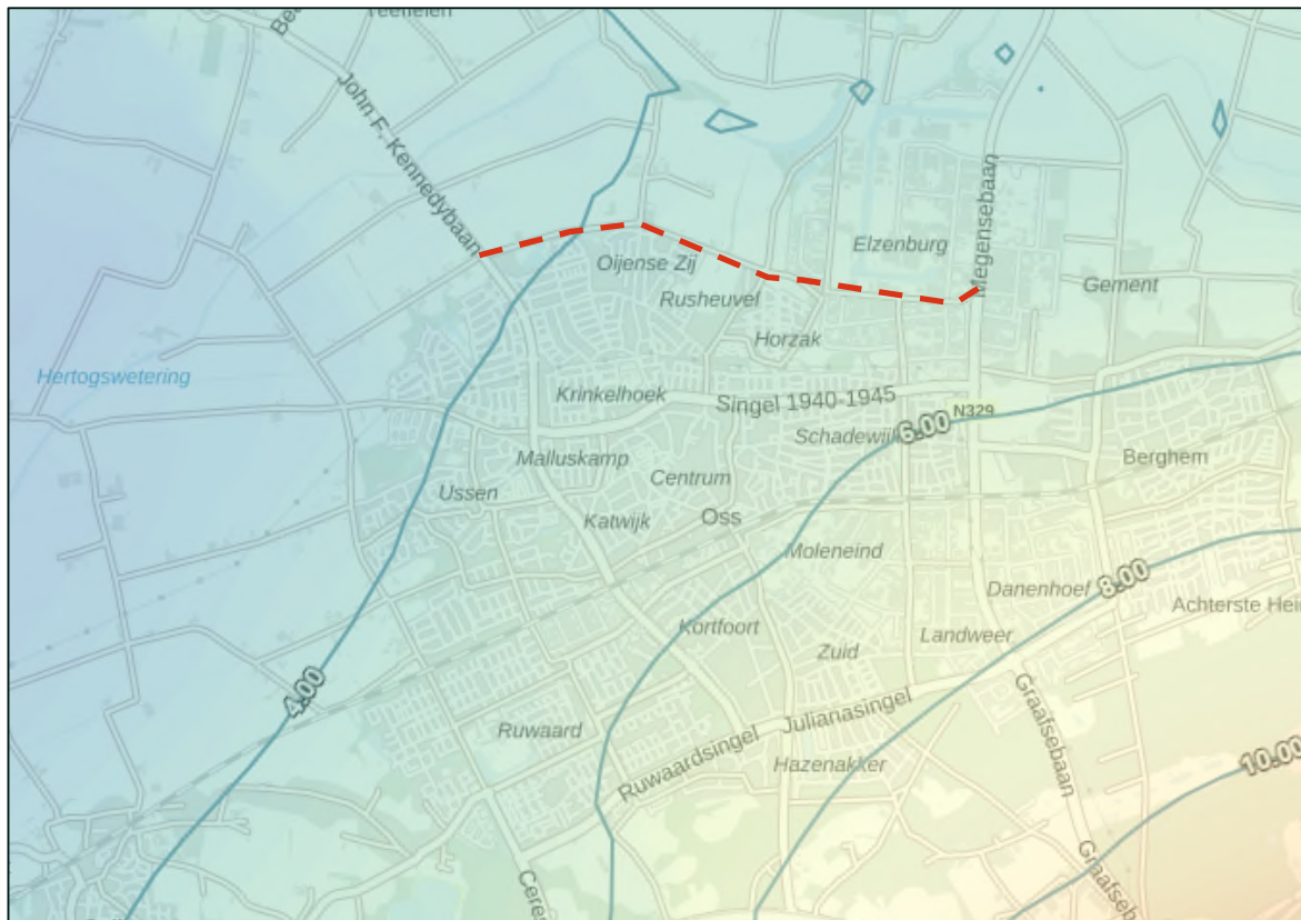
Figuur 2-6 Uitsnede isohypsenkaart LHM laag 1, projectlocatie Oss. Gemiddelde grondwaterstand (metingen 2019) [NAP m.] Uitgaande van een gemiddeld maaiveld niveau van NAP +5 in het westen tot NAP +6,5 m in het oosten wordt de grondwaterstand op circa 1 à 1,5 m -mv. verwacht.
