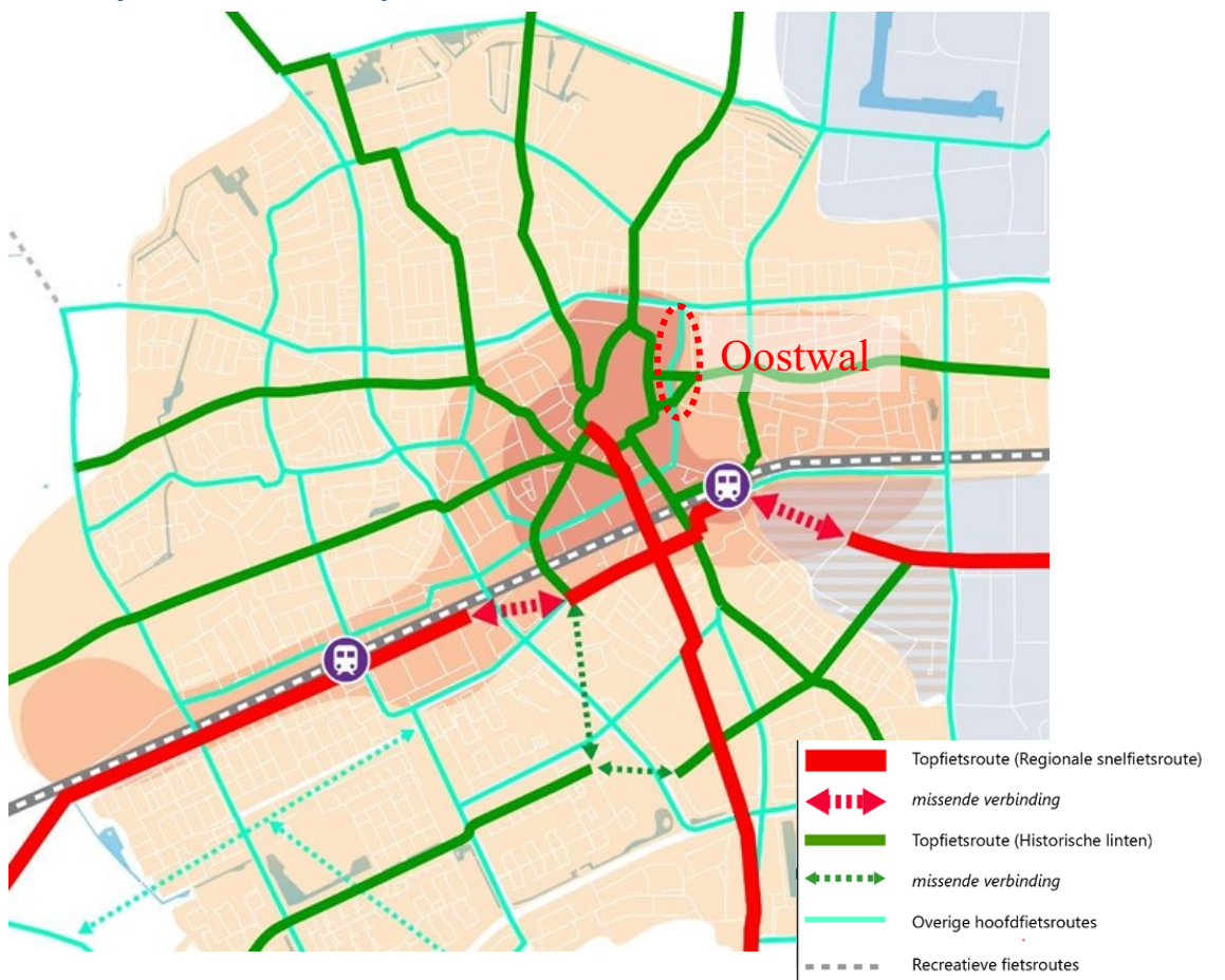
Hoofdstructuur fiets
