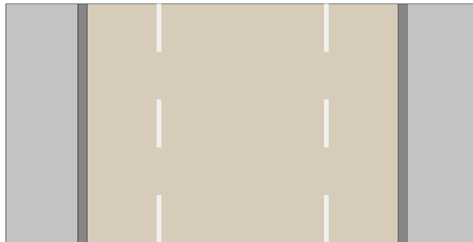
Dwarsprofiel: Erftoegangsweg Type I binnen bebouwde kom
