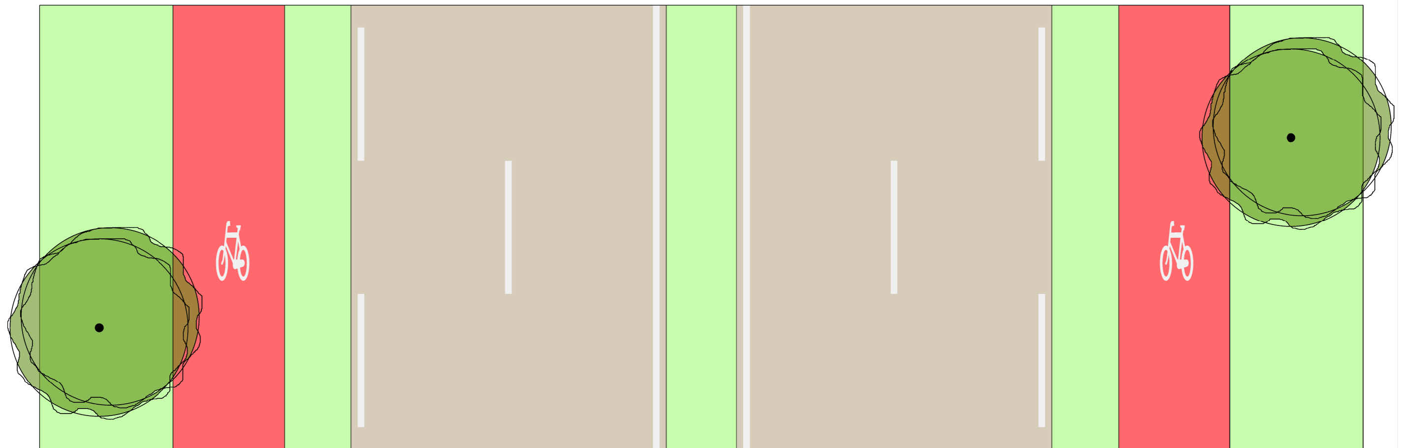
Dwarsprofiel: Gebiedsontsluitingsweg 70 km/h 2x2 binnen bebouwde kom
