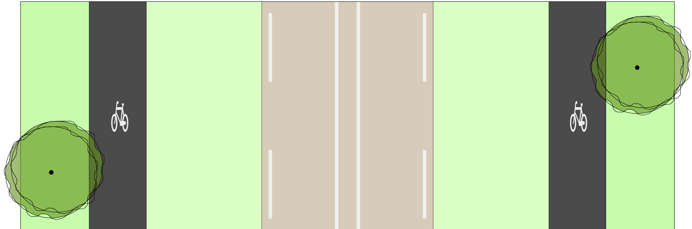
Dwarsprofiel: Gebiedsontsluitingsweg Type II 80 km/h buiten bebouwde kom
