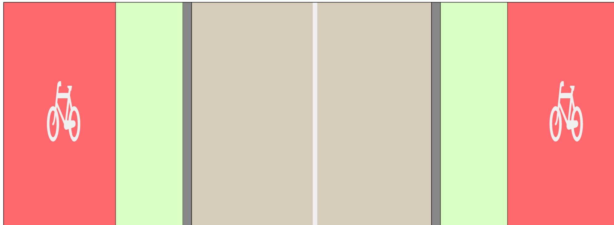
Dwarsprofiel: Gebiedsontsluitingsweg 50 km/h Type I binnen bebouwde kom
